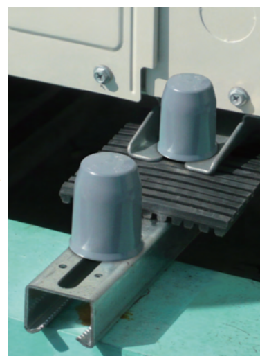
施工後
