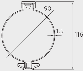
構造図 (単位:mm)
