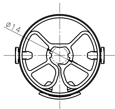
A矢視図
