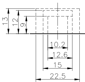
適合:1~4号 側面ロックアウトA詳細図(1:1)
