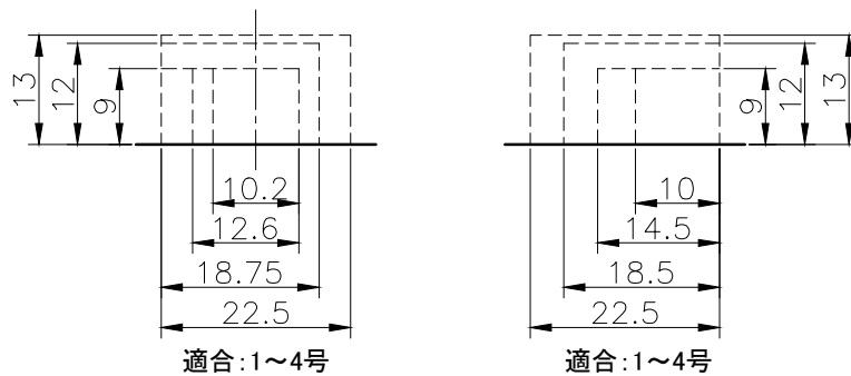
側面ノックアウトA詳細図(1:1) 側面ノックアウトB詳細図(1:1)
