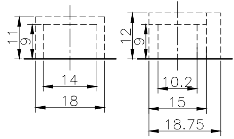
浅型 適合:1,2号 深型 適合:1~3号 側面ロックアウトA詳細図(1:1)
