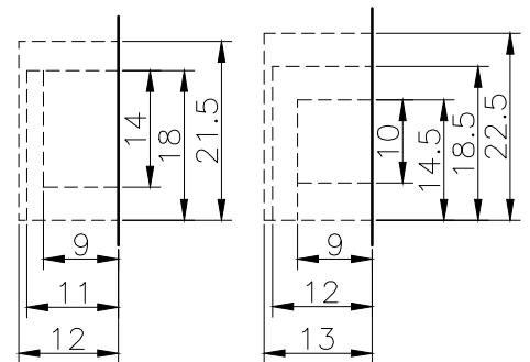
浅型 適合:1~3号 深型 適合:1~4号 側面ロックアウトC詳細図(1:1)
