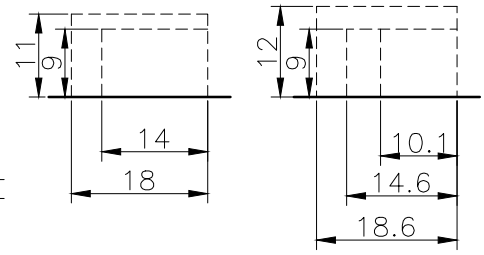
浅型 適合:1,2号 深型 適合:1~3号 側面ロックアウトB詳細図(1:1)
