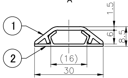
2号 A矢视图
