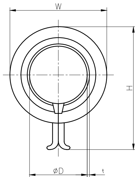
A矢视图(1:2)
