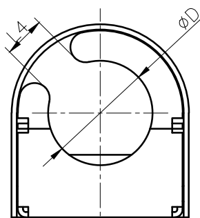
A矢视图
