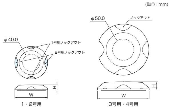
寸法表
