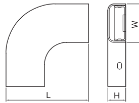
■規格表
