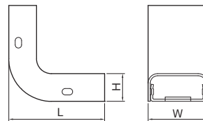
■規格表
