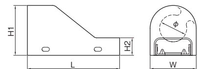
寸法表
