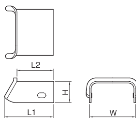
寸法表
