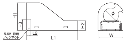
寸法表
