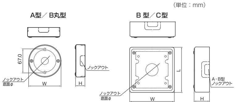
寸法表
